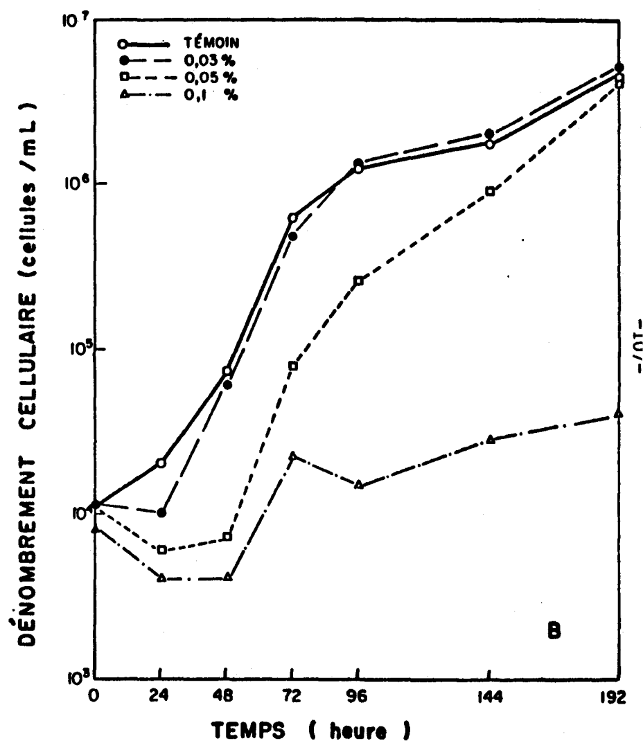
Figure 9: Récupération des algues en milieu sain après (a) 24 heures d'exposition, et (b) 48 heures d'exposition.
