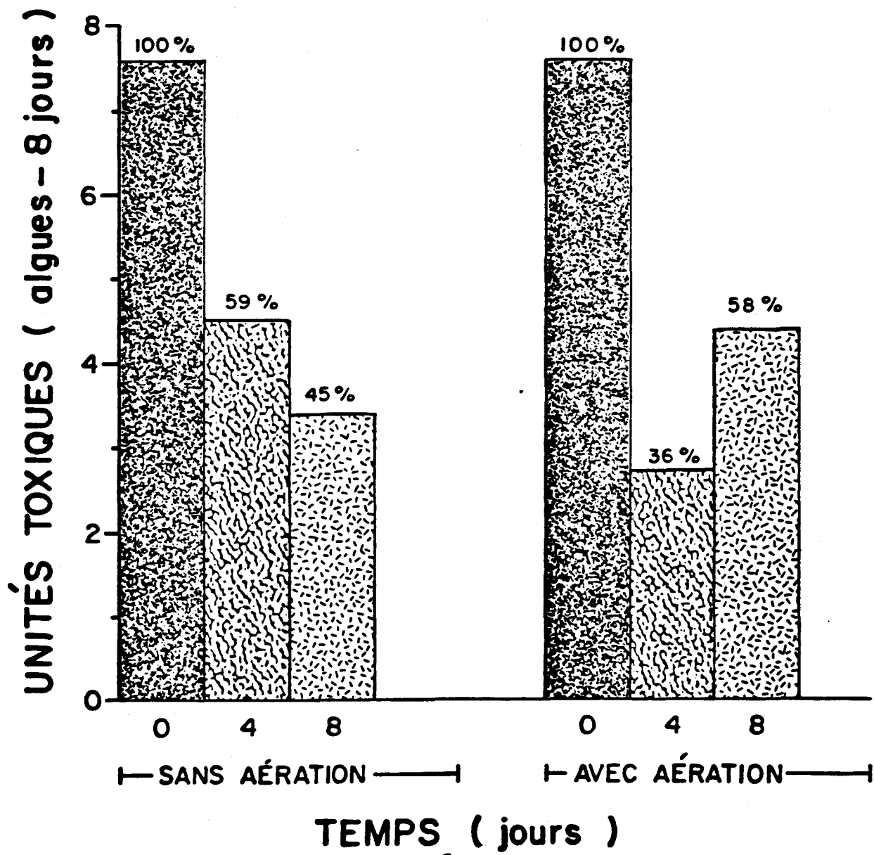
Figure 3: Profil de la réduction de toxicité (test algal - 8 jours) pendant le vieillissement de l'effluent de pâtes et papiers utilisant les procédures sans et avec aération. Les pourcentages font référence à la toxicité du jour 0.
