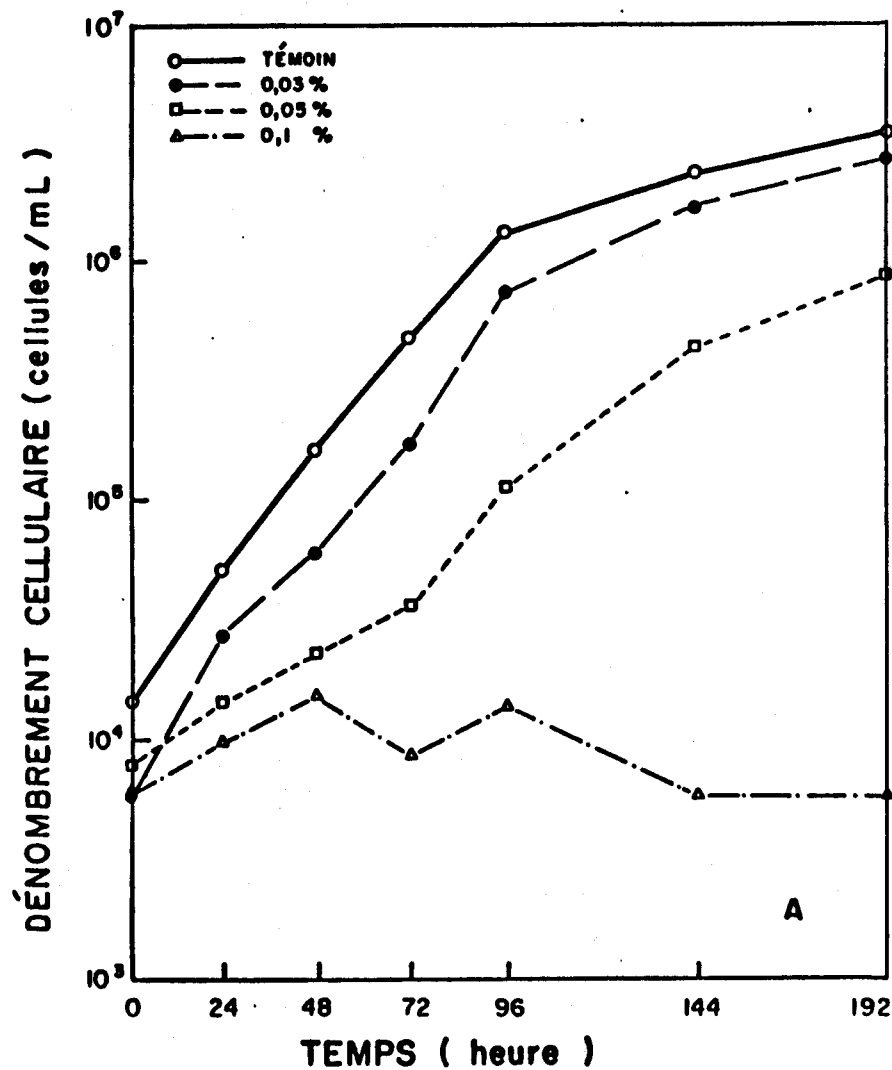
Figure 11: Courbes de croissance des algues repiquées en milieux contaminés après (a) 96 heures de pré-exposition et (b) 192 heures de pré-exposition.
