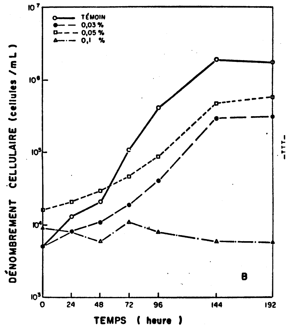
Figure 11: Courbes de croissance des algues repiquées en milieux contaminés après (a) 96 heures de pré-exposition et (b) 192 heures de pré-exposition.
