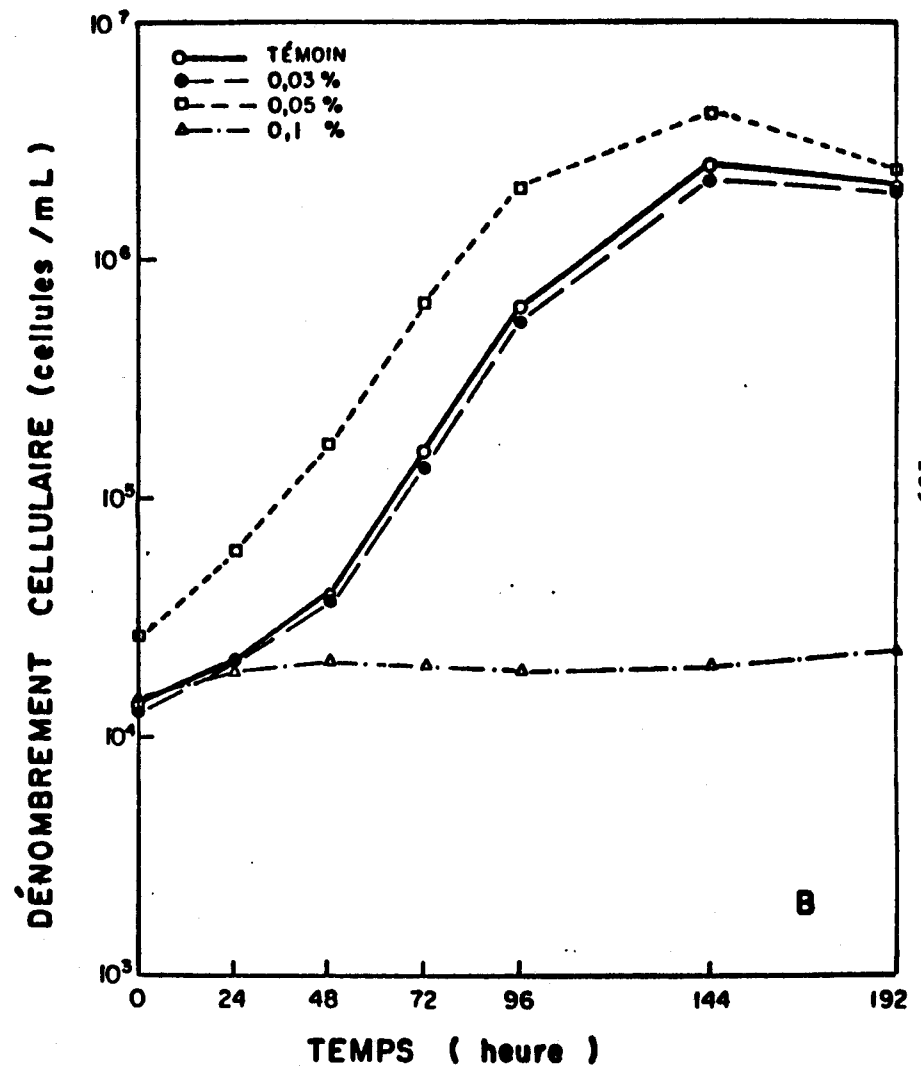
Figure 10: Récupération des algues en milieu sain après (a) 96 heures d'exposition et (b) 192 heures d'exposition.
