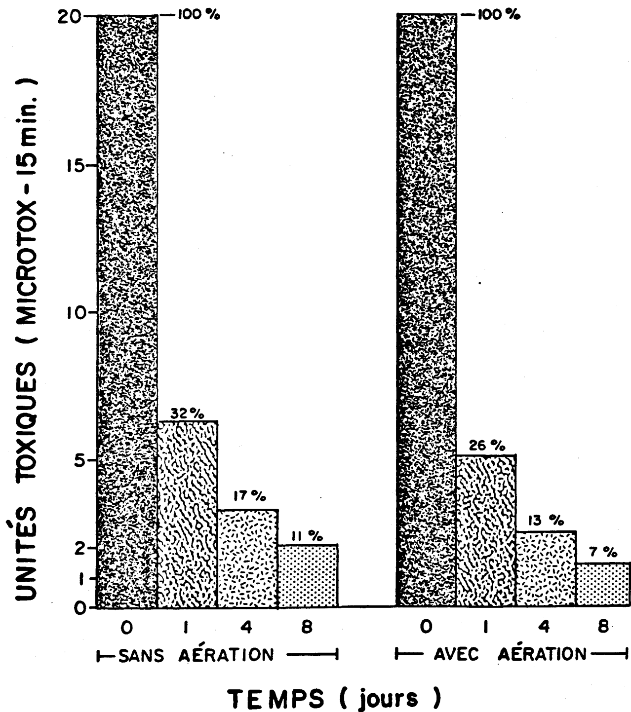
Figure 2: Profil de réduction de la toxicité (Microtox - 15 min.) pendant le vieillissement de l'effluent de pâtes et papiers, utilisant les procédures sans et avec aération. Les pourcentages font référence à la toxicité du jour 0.
