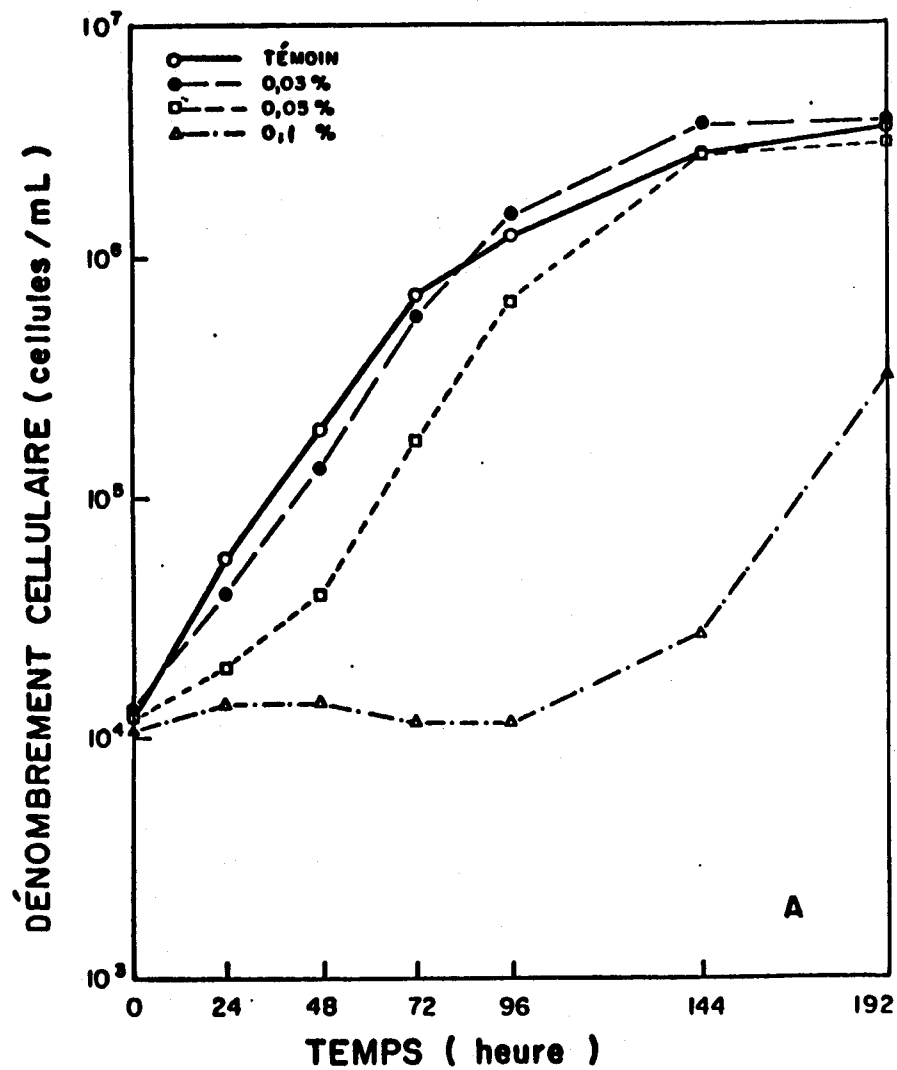
Figure 10: Récupération des algues en milieu sain après (a) 96 heures d'exposition et (b) 192 heures d'exposition.
