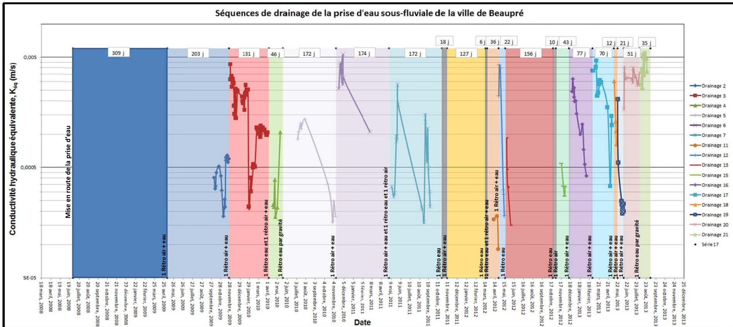
Figure 2 : Séquences de drainage de la prise d'eau sous-fluviale de Beaupré : valeurs de conductivité hydraulique équivalente lors des séquences de drainage
