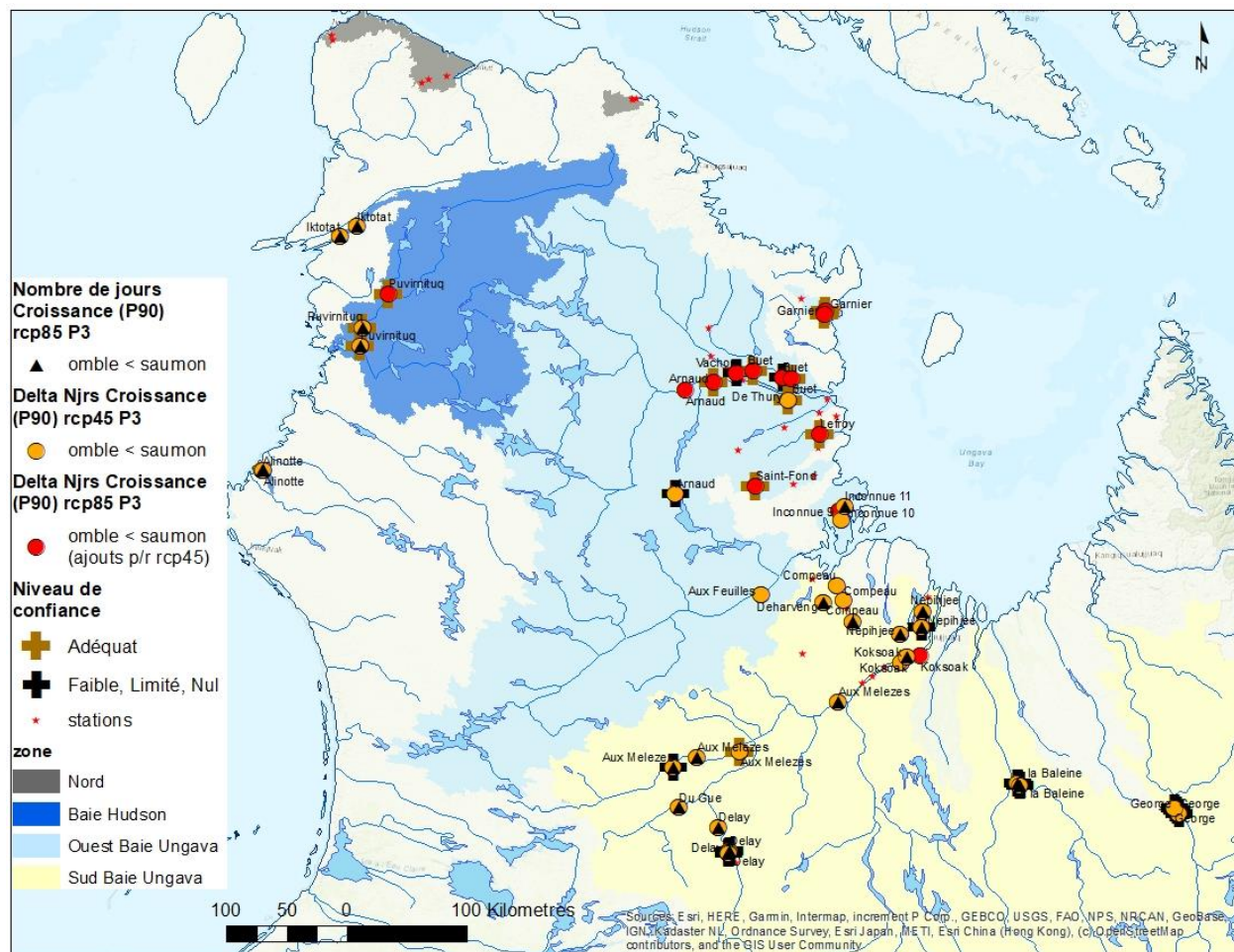
Figure 39. Distribution spatiale des stations pour lesquels le nombre de jours de croissance optimale et le delta de changements de ce nombre sont inférieurs pour l'omble chevalier que pour le saumon à la période 2071-2100 et pour les scénarios rcp4.5 et rcp8.5. Les triangles noirs indiquent les stations où le nombre annuel moyen de jours de croissance optimale pour le saumon est supérieur à celui pour l'omble chevalier. a) les résultats obtenus avec la moyenne des modèles climatiques; b) les résultats obtenus avec P90 des modèles climatiques. Pour simplifier la carte, les niveaux de confiance « faibles », « limité » et « nul » sont représentés par un même symbole et les niveaux « modérés » et « bon » ne sont pas représentés. Le nom de la rivière associée à chacune des stations est inscrit. Les stations où le nombre annuel moyen de jours de croissance optimale et le delta de changements à la période 2071-2100 sont supérieurs pour l'omble chevalier que pour le saumon sont identifiées par une petite étoile rouge.
