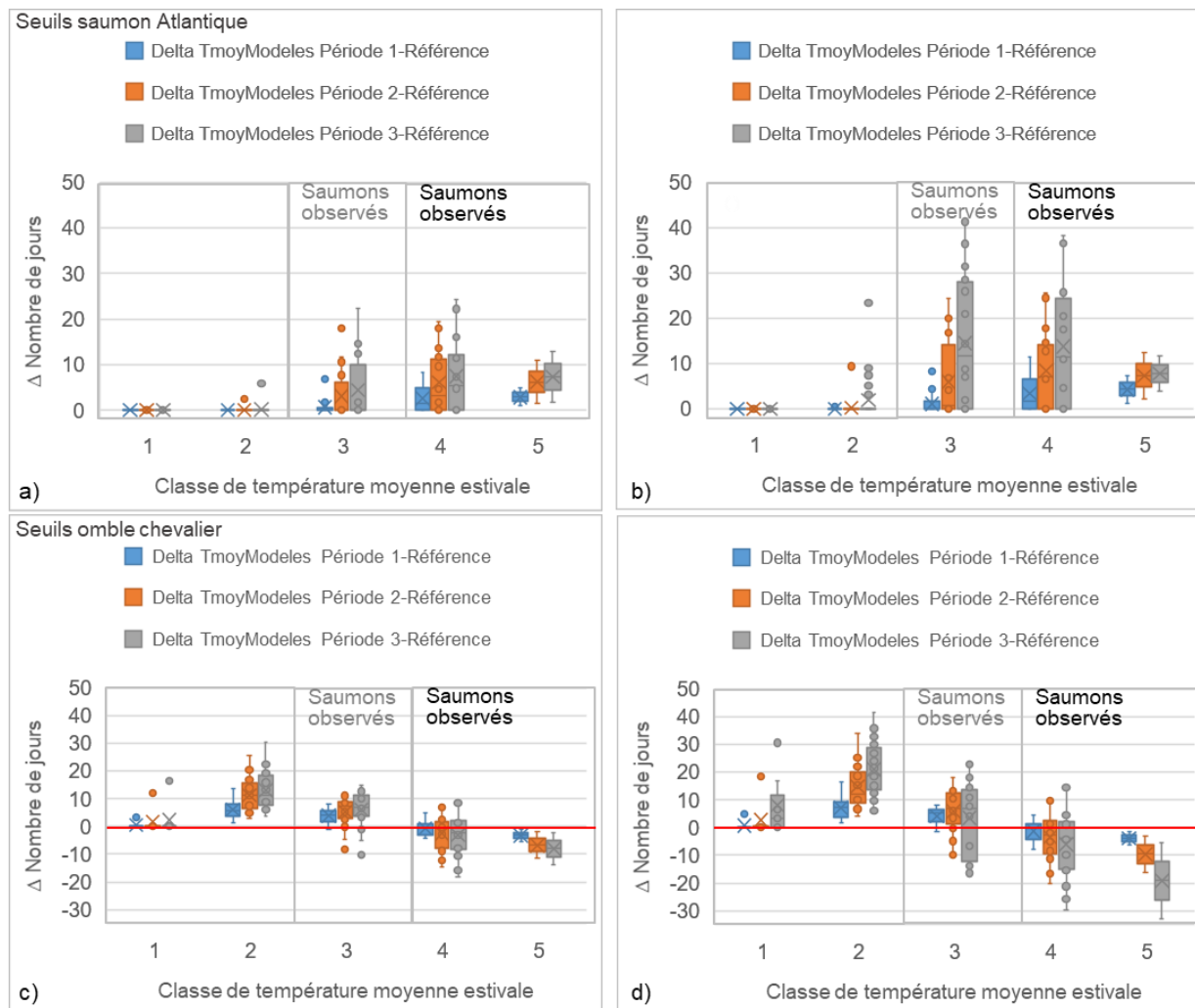
Figure 37. Delta de changement du nombre annuel moyen de jours de croissance optimale (moyenne de modèles climatiques) en fonction des classes de la moyenne estivale de Teau moy (période de référence). a) Pour le saumon rcp4.5 et b) Pour le saumon rcp8.5; c) Pour l'omble chevalier rcp4.5 et d) Pour l'omble chevalier rcp8.5. Classe 1: 6^{\circ}\text{C} < T < 8^{\circ}\text{C} ; Classe 2: 8^{\circ}\text{C} < T < 10^{\circ}\text{C} ; Classe 3: 10^{\circ}\text{C} < T < 12^{\circ}\text{C} ; Classe 4: 12^{\circ}\text{C} < T < 14^{\circ}\text{C} ; Classe 5: 14^{\circ}\text{C} < T < 16^{\circ}\text{C} . Les deltas sont calculés par rapport à la période de référence. Les saumons sont observés dans les rivières des classes 4 et 5 et dans 3 des 12 rivières de la classe 3.
