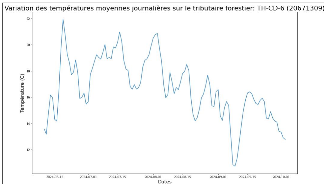
Figure B7. Variation des températures moyennes journalières sur la tributaire forestier, jauge en été 2024.
