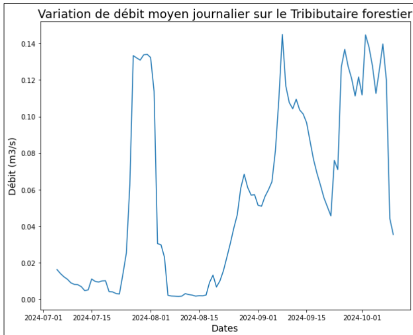
Figure B6. Variation du débit moyen journalier sur le tributaire forestier, jaugé en été 2024.
