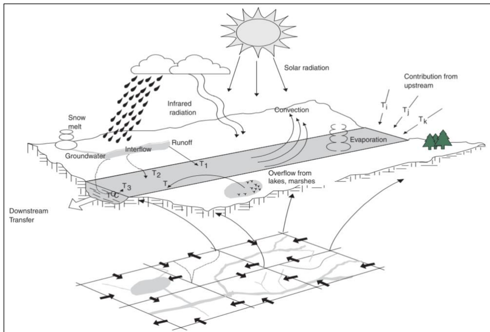
Figure 2. Représentation des composantes du bilan thermique inclus dans le modèle de température d'eau du CEQUEAU (Morin and Couillard, 1990; St-Hilaire et al., 2011).
