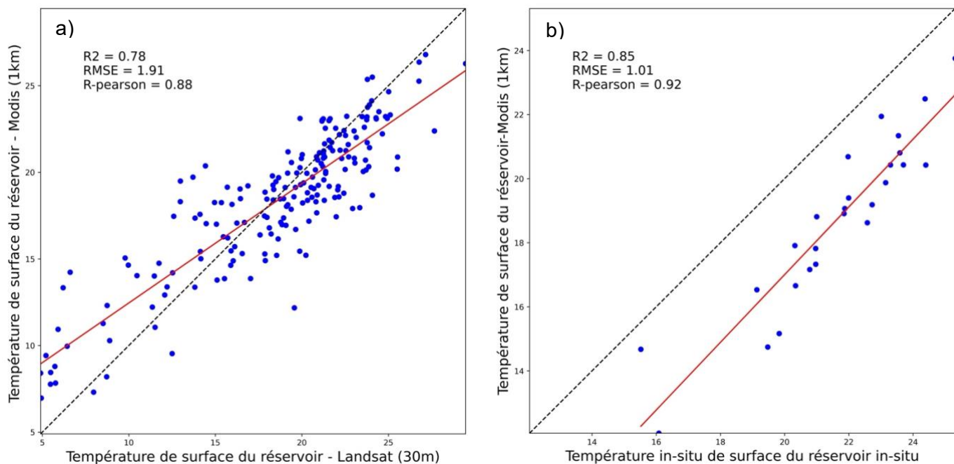
Figure 9. Validation des températures de surface de MODIS par rapport (a) aux températures de surface du LANDSAT (30 m) et (b) aux mesures in-situ prises en été 2024.
