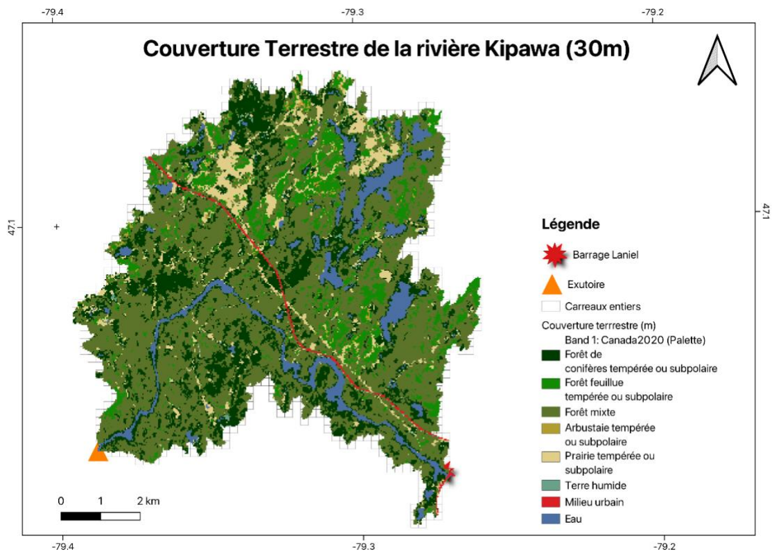
Figure B4. Couverture terrestre du bassin versant Kipawa, divisé en carreaux entiers.
