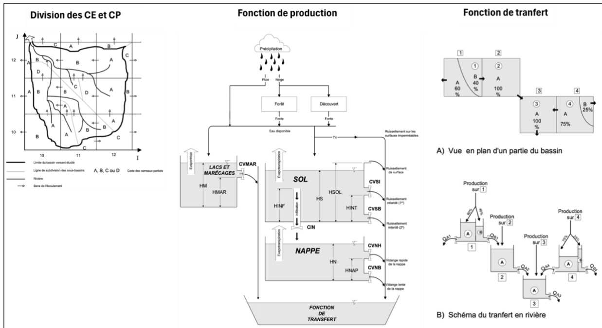
Figure B1. Principe de la modélisation hydrologique dans CEQUEAU (André St-Hilaire et al. 2011; Morin et Paquet 1995).
