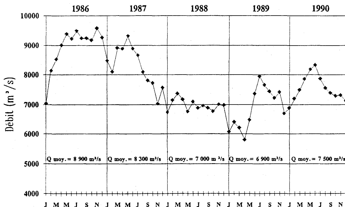
Figure 7 - Hydrogramme du fleuve Saint-Laurent pour le secteur de Cornwall-Massena (1986 à 1990)
