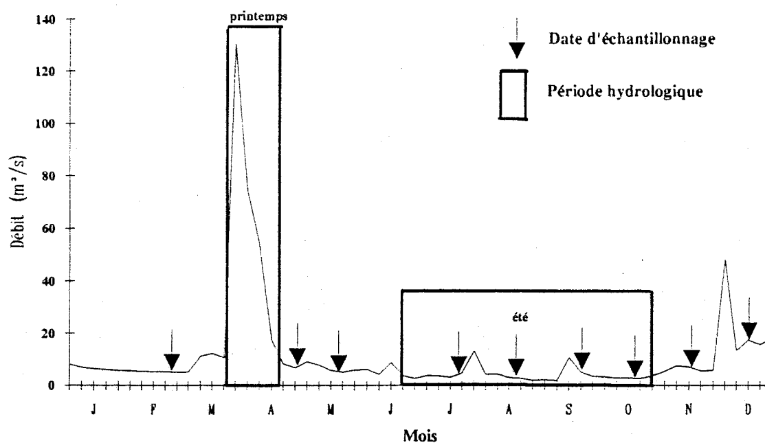
Figure 4 - Saisons printanière et estivale représentées sur l'hydrogramme de la rivière aux Saumons à l'embouchure pour l'année 1987
