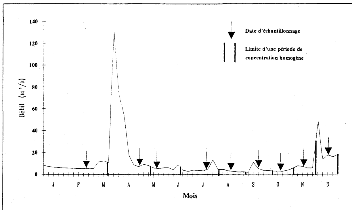
Figure 3 - Périodes de concentration homogène représentées sur l'hydrogramme de la rivière aux Saumons à son embouchure pour l'année 1987
