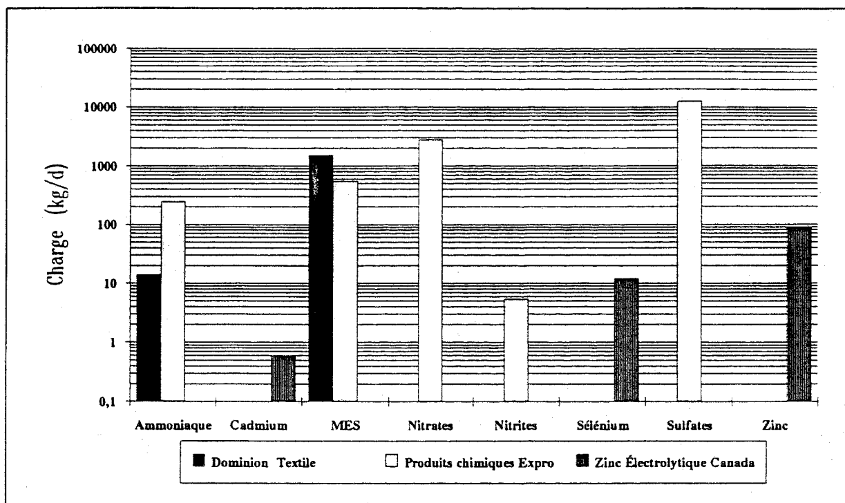
Figure 2 - Charges journalières (kg/d) des principaux contaminants industriels du tronçon Cornwall-Beauharnois (ZIP 3 et 4 uniquement)
