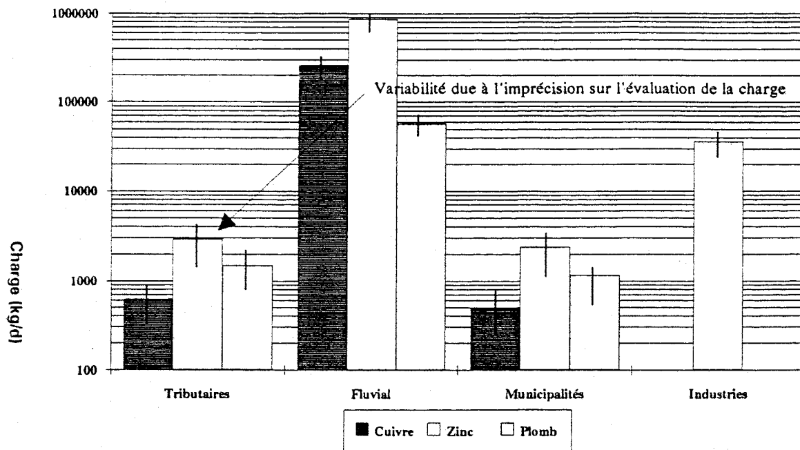
Figure 9 - Bilan de charge pour les trois métaux de référence des quatre principales sources de contamination du tronçon Cornwall-Beauharnois.
