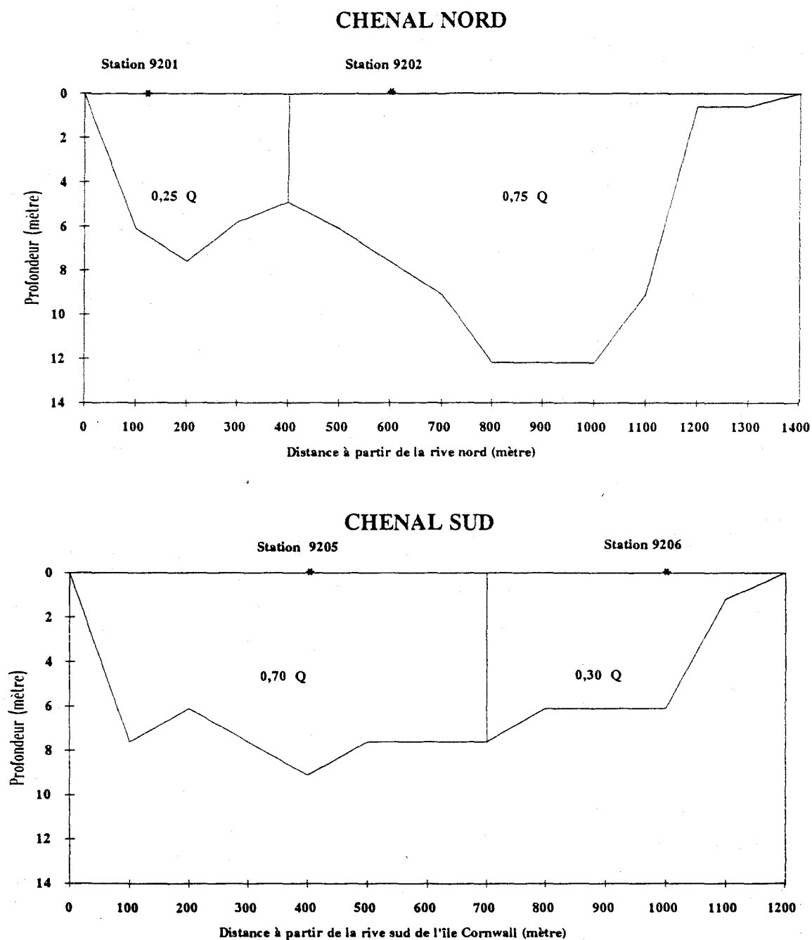
Figure 8 - Profils bathymétriques des chenaux nord et sud du fleuve Saint-Laurent et localisation des stations de mesure de qualité de l'eau au transect de Cornwall
