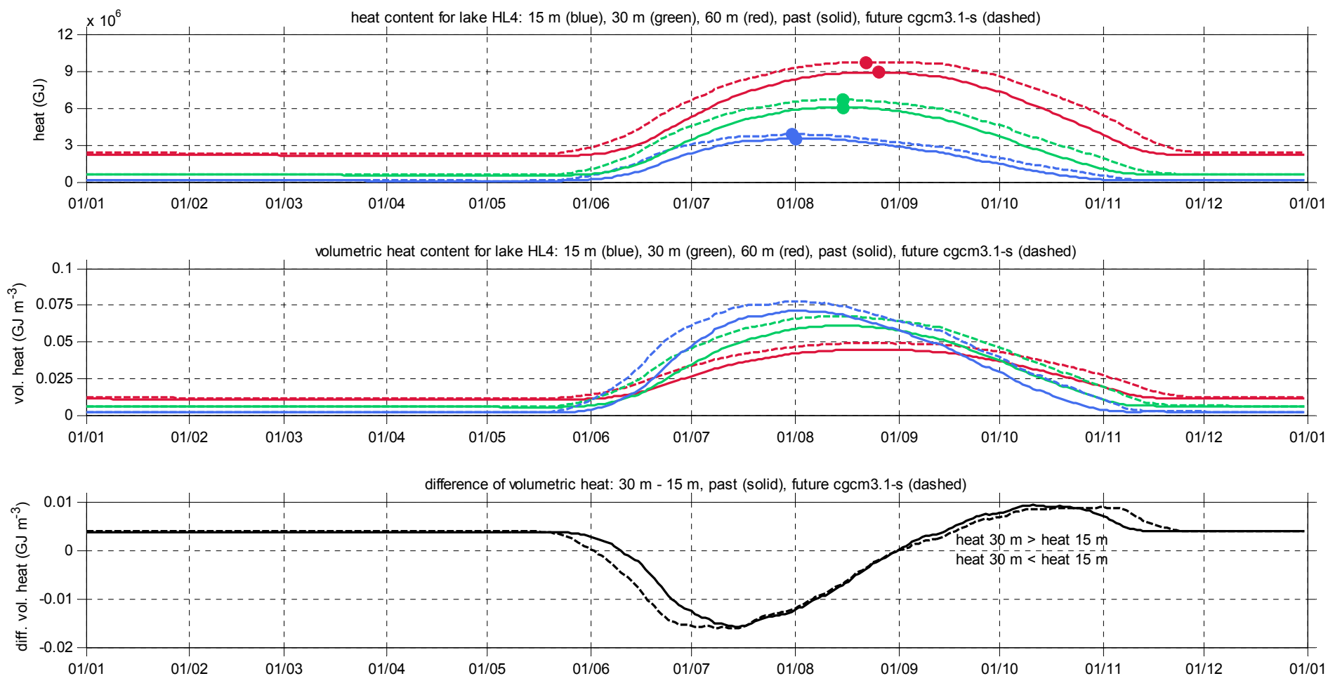
Figure 5.5.2 En haut : cycle annuel de contenu en chaleur passé (lignes continues) et futur (lignes pointillées) pour trois lacs hypothétiques de différentes profondeurs (15 m, bleu; 30 m, vert; 60 m, rouge) à la latitude HL4. Les points indiquent l'occurrence des maximums. Au milieu : idem pour contenu en chaleur volumique. En bas : différence de contenu en chaleur volumique « lac 30 m-lac 15 m » passée (ligne continue) et future (ligne pointillée). Les contenus en chaleur futurs sont obtenus de la moyenne des simulations pilotées par le modèle global CGCM3.1.
