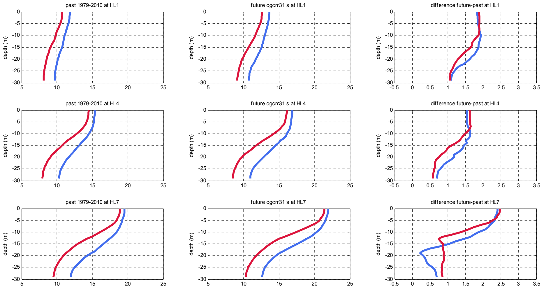
Figure 5.5.6 Profils de température passée et future pour la période 11-20 août pour deux lacs hypothétiques de volume différent ( 0,10 \text{ km}^3 , bleu; 0,15 \text{ km}^3 rouge) lorsque placés aux latitudes HL1, HL4 et HL7, et différences « futur-passé ». Les températures futures 2041-2070 sont obtenues de la moyenne des simulations pilotées par le modèle global CGCM3.1.
