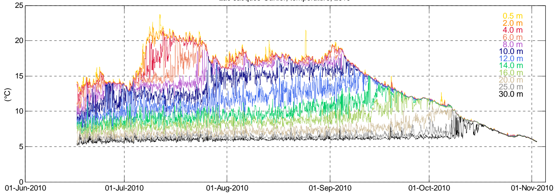
Lac Jacques-Cartier, température, 2010
