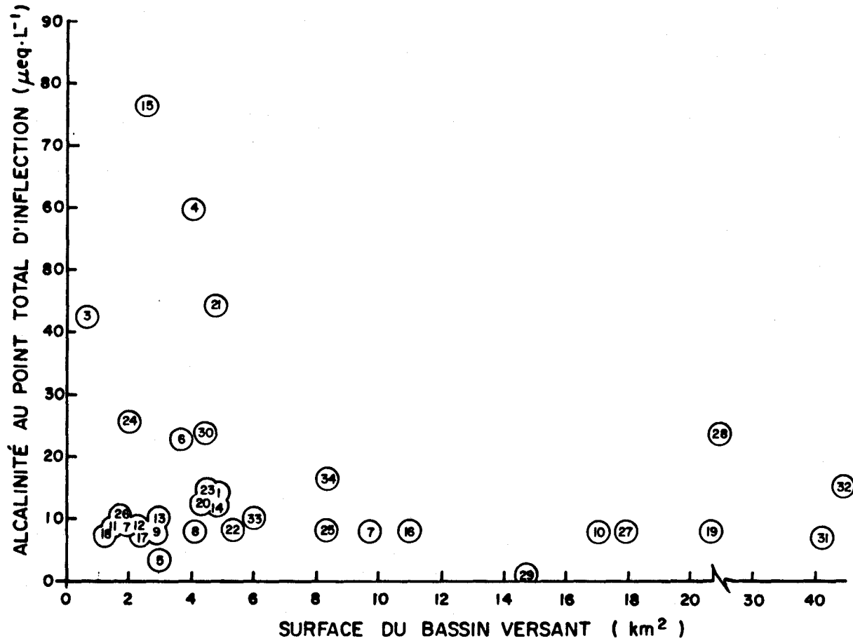
FIGURE C1 Relation entre l'alcalinité au point total d'inflection ( \mu \text{ eq.L}^{-1} ) versus surface du bassin versant ( \text{km}^2 ).
