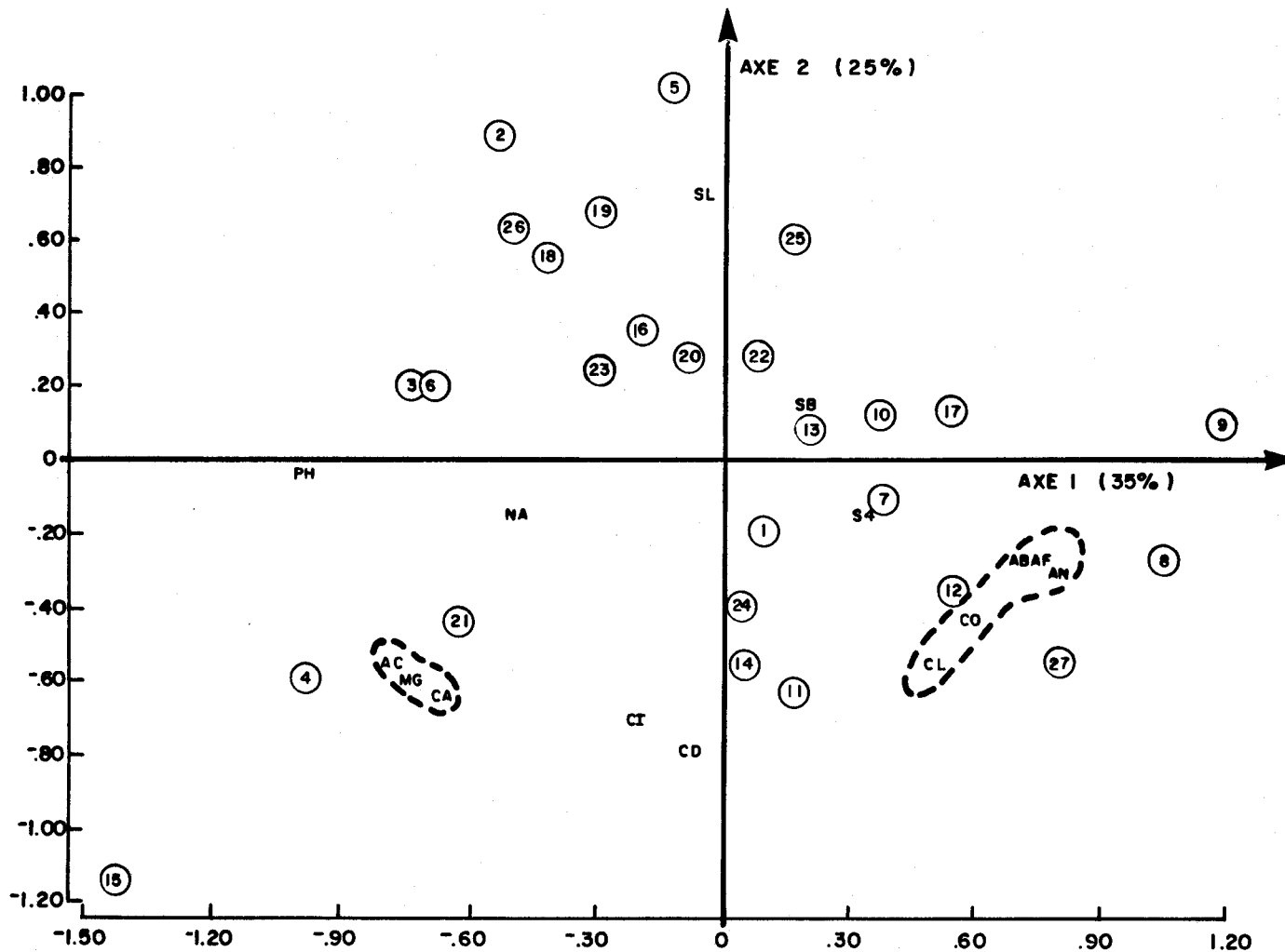
FIGURE 9 Projection des deux premiers axes de l'analyse en composantes principales effectuée sur la matrice du tableau 2. Symbolisme: voir figure 8.
