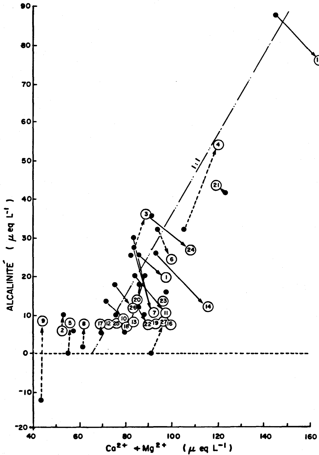
FIGURE 3 Graphique de l'alcalinité ( \mu \text{ éq.L}^{-1} ) versus [\text{Ca}^{2+} + \text{Mg}^{2+}] ( \mu \text{ éq.L}^{-1} ). Distribution des lacs échantillonnés le 19.11.80.
