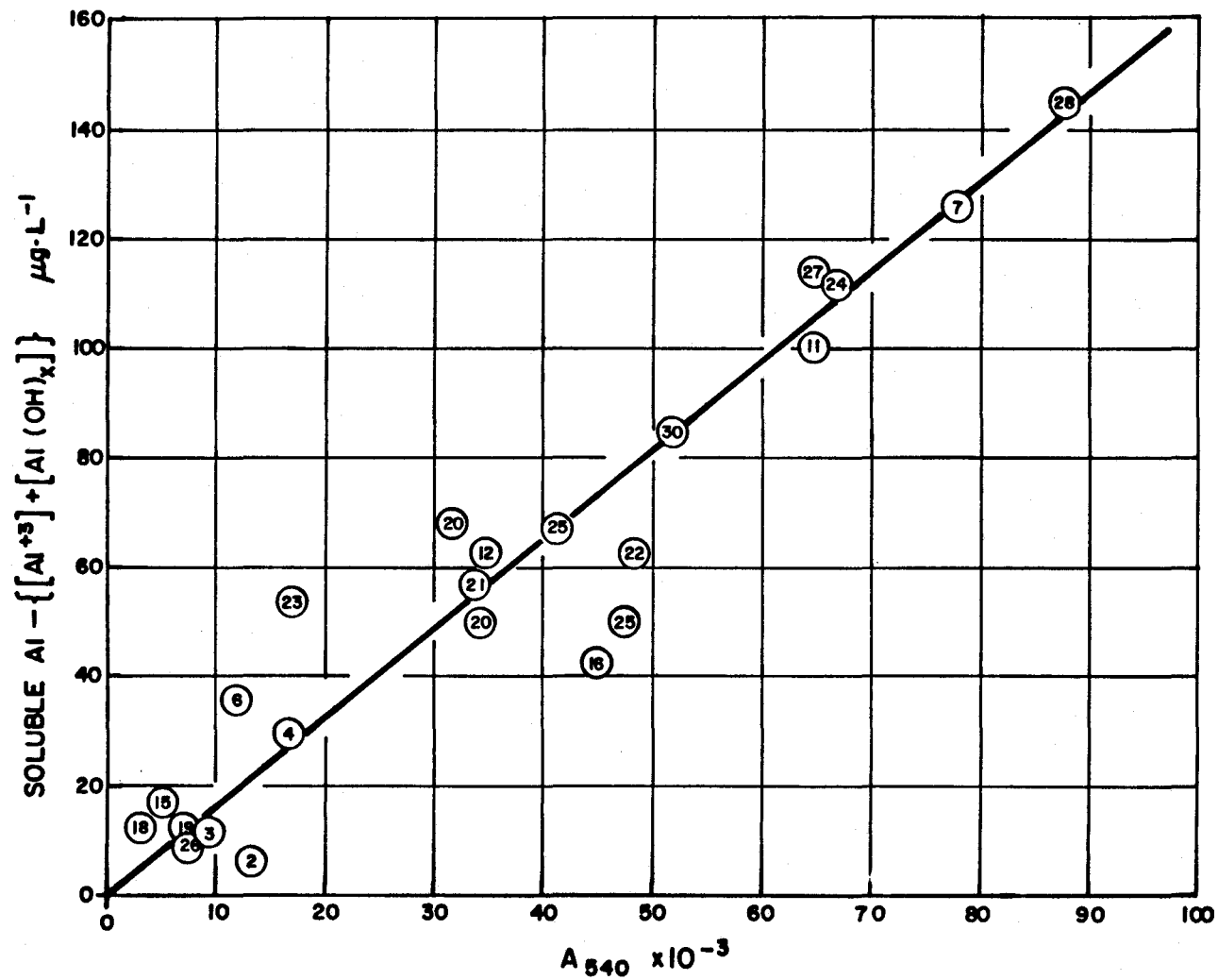
FIGURE 14 Graphique de l'aluminium soluble - [\text{Al}^{3+}] + [\text{Al}(\text{OH})_x] ( \mu\text{g}\cdot\text{L}^{-1} ) versus absorbance à 540 nm. Chiffres = distribution des lacs.
