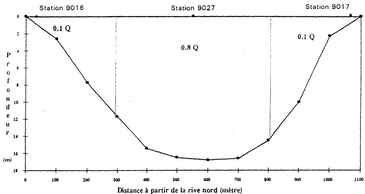
Figure 8 - Profil bathymétrique du fleuve Saint-Laurent et localisation des stations de mesures de qualité de l'eau au transect de Lanoraie
